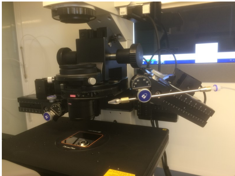
Pant pro vertikální vyklápění mikromanipulátoru
