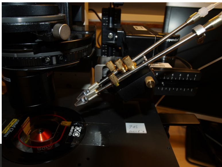
Držák dvou kapilár (Synga)
